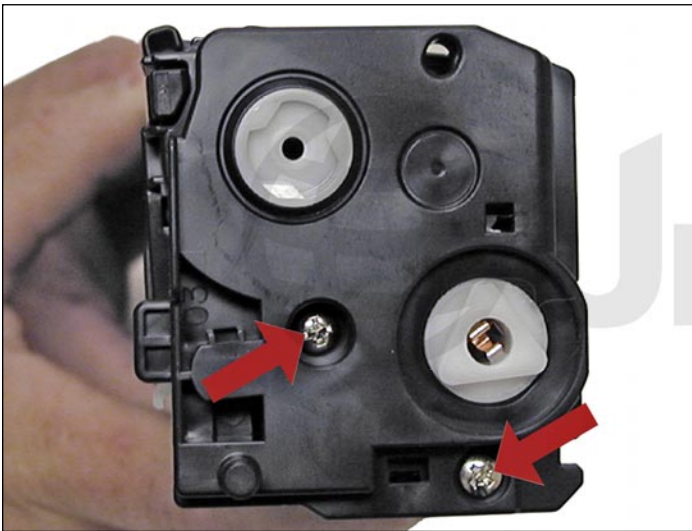
27. Instale la cubierta lateral exterior del lado del engranaje y los dos tornillos.
