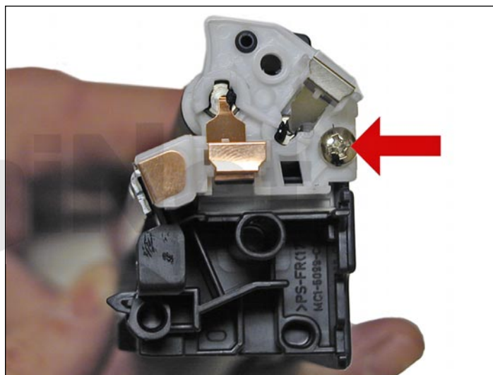
22. Reemplace la cubierta lateral de contacto y el tornillo.
