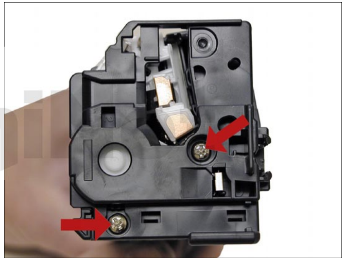
28. Instale la cubierta lateral exterior restante en el lado de contacto del cartucho y los dos tornillos.
