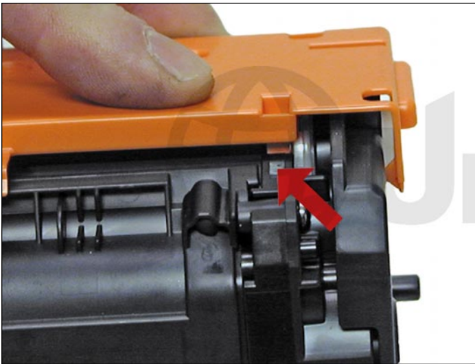
29. Instale la cubierta del cilindro en el cartucho.
