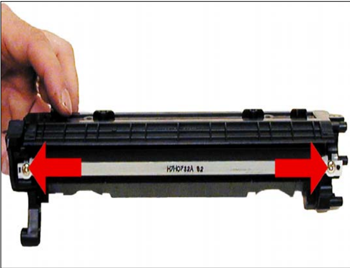
21. Montar la cuchilla dosificadora con sus dos tornillos.
