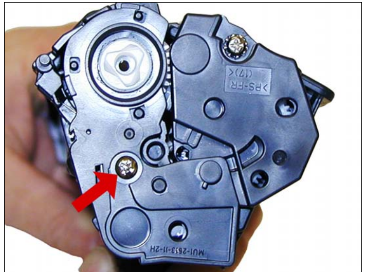
28. Levantar el extremo del resorte para fijarlo a la tapa de OPC como se muestra. Fijar el tornillo a la tapa.
